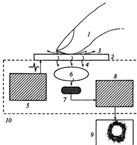
Рис. 2. Схематическое изображение ГРВ-прибора. 1 – объект исследования; 2 – прозрачный электрод; 3 – газовый разряд; 4 – оптическое излучение; 5 – генератор; 6 – оптическая система; 7, 8 – видеоспреобразователь; 9 – компьютер; 10 – корпус.
